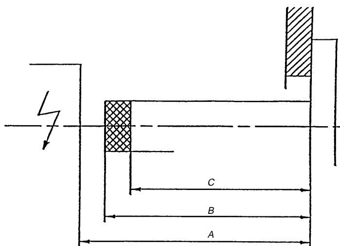
Figure A.2 – Gamme de tolérances sur la longueur d'un calibre d'essai
